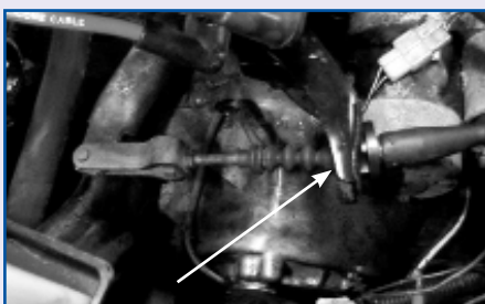
Clutch cable seizure
